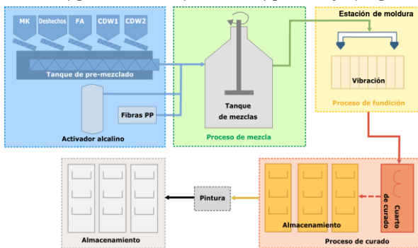
Esquema de la Planta Piloto de Mejora de la Tecnología
