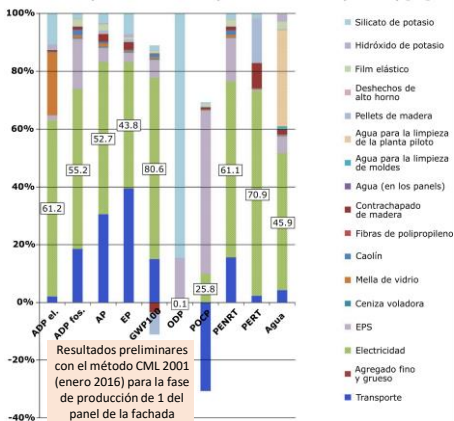
Resultados preliminares con el método CML 2001 (enero 2016) para la fase de producción de 1 del panel de la fachada (0.36 m 2 ) [%]
