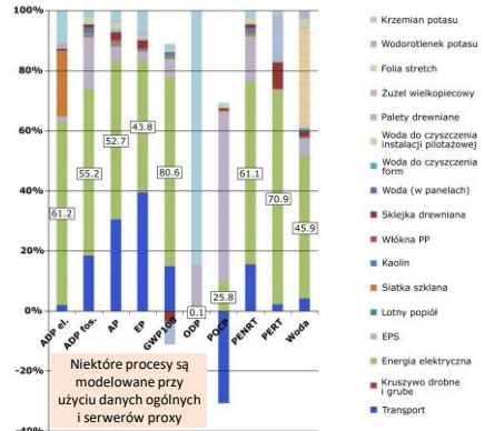
Wstępne wyniki z zastosowaniem metody CML 2001 (sty. 2016 r.) na etapie produkcji panelu elewacyjnego (0.36 m 3 ) [%]
