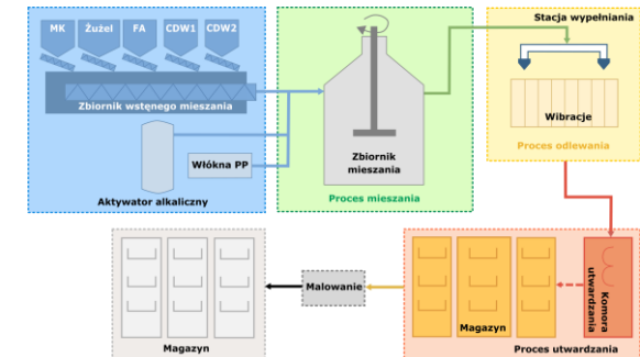
Schemat „Pilotażowego Zakładu Skalowania Technologii”
